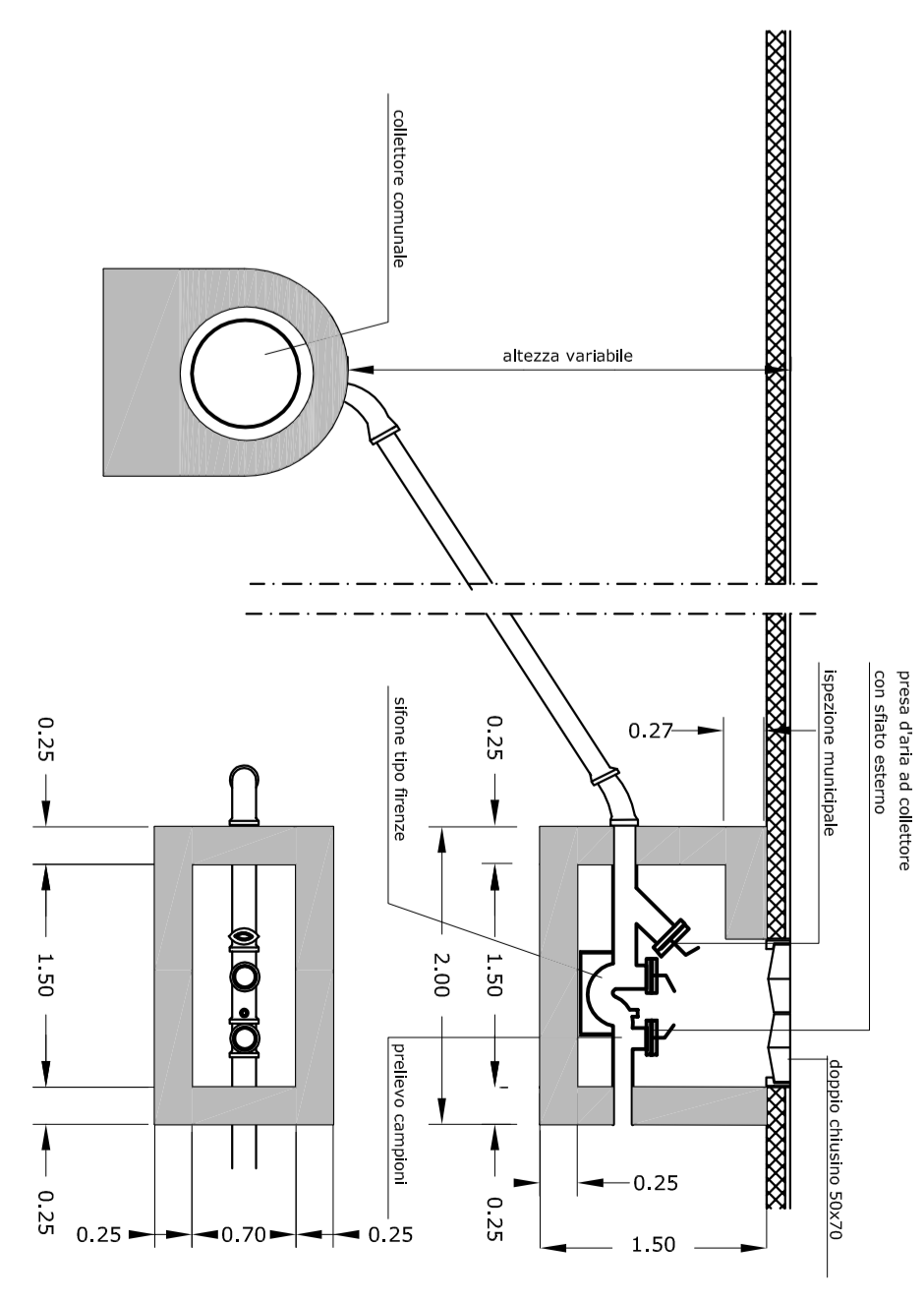
Allacciamento tipo alla fognatura comunale
